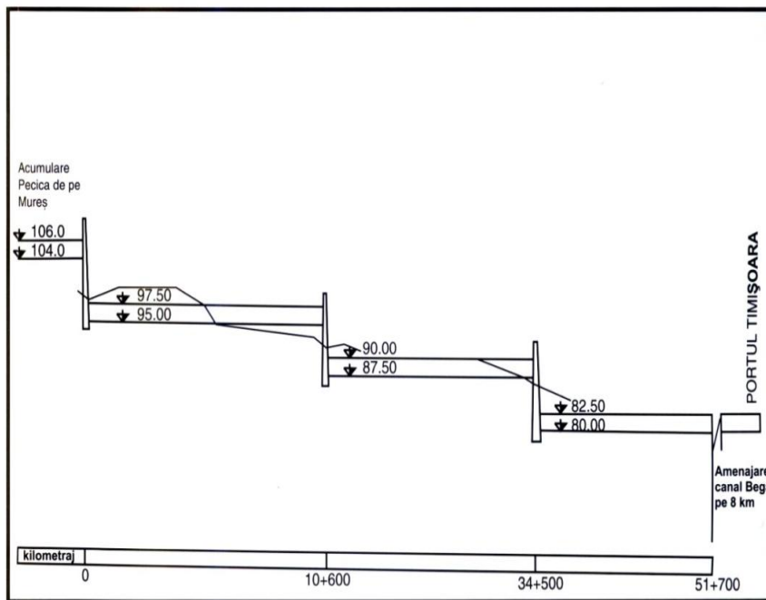
Schema hidrotehnica
